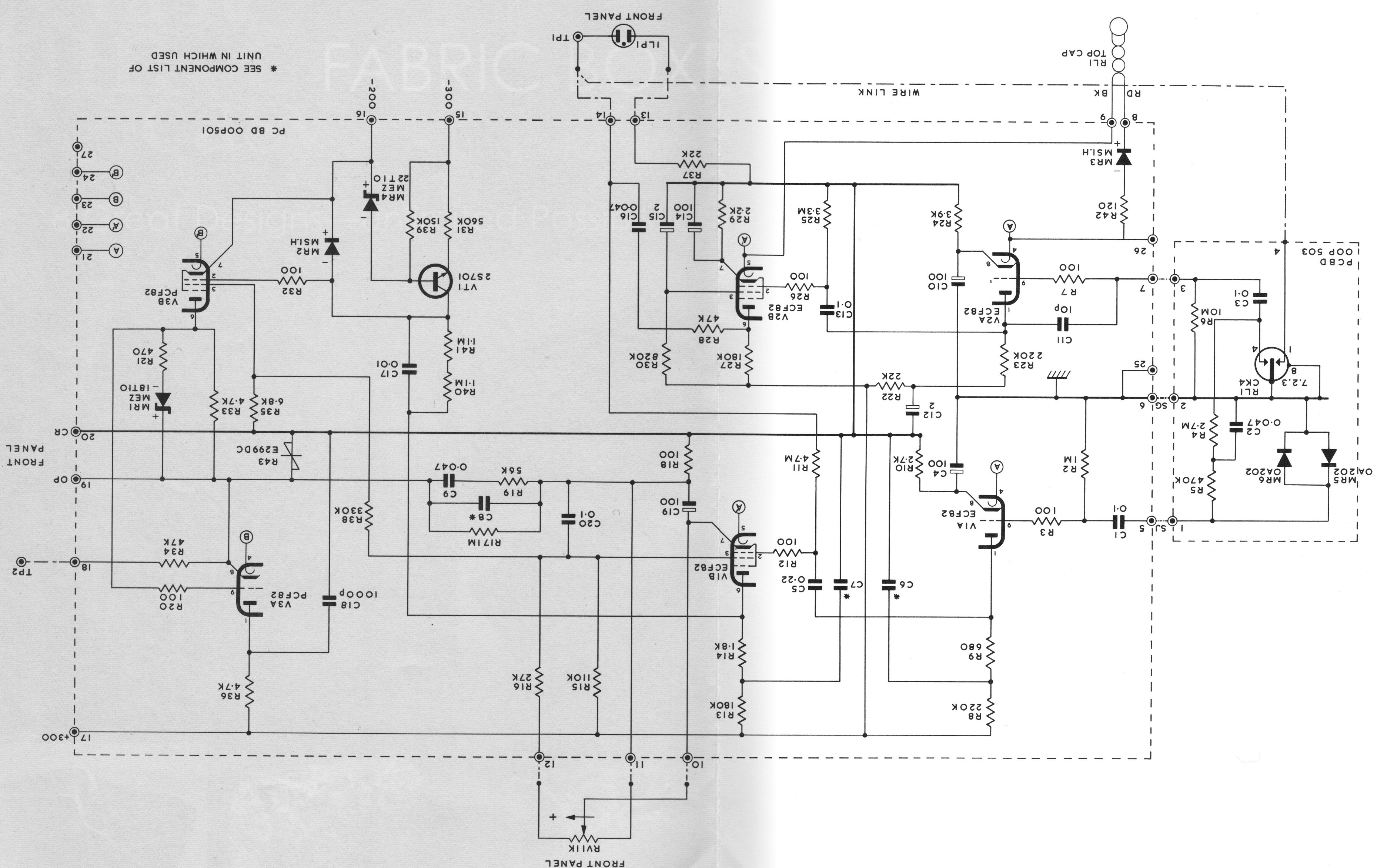
Fig. 3 - Circuit Diagram : OOP501/503
